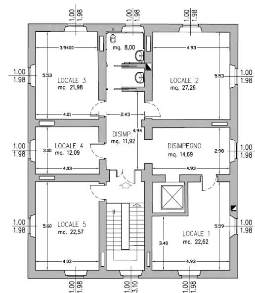
PIANO SECONDO H 3.50
